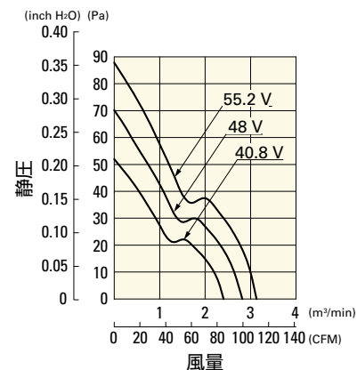
9WP1248H101 バルスセンサ付
