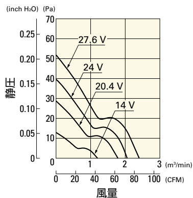
9WP1224M101 バルスセンサ付
