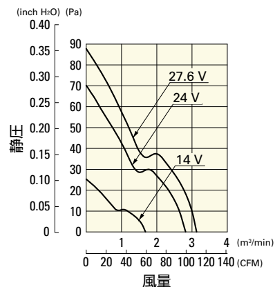
9WP1248M101 バルスセンサ付
